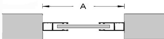
SISTEMA C: CON GUIAS EN SUPERFICIE
