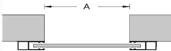
SISTEMA B: CON GUIAS SOLAPADAS
